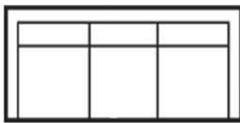
3 Seater Settee H:97cm W:206cm D:97cm
